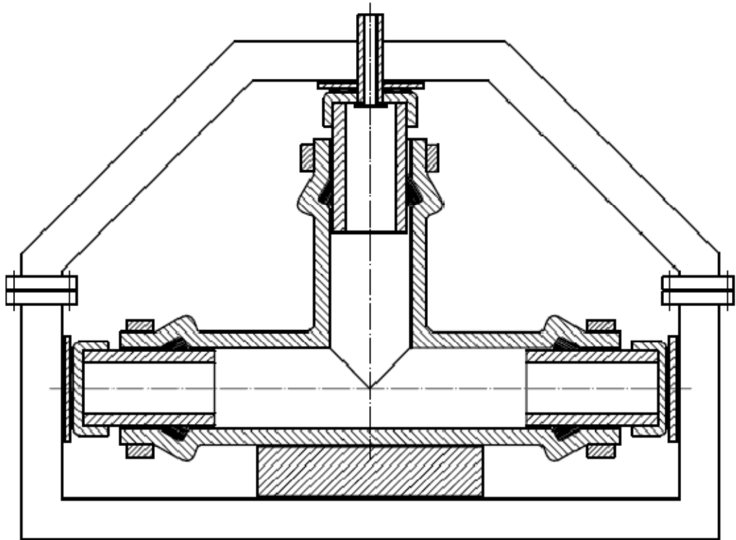
شکل ۶- مثالی از آزمون‌های فشار بند، با استفاده از وسایل درگیر با قاب بیرونی، و بدون فشار محوری هیدرواستاتیک
